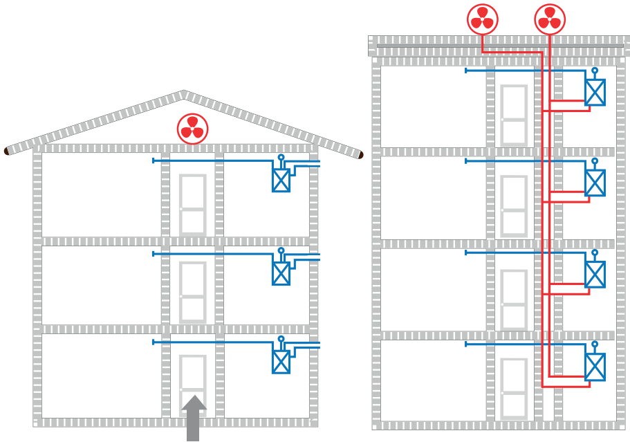
PluggPlan Lüftungssystem einheitszentral mit Schachtführung und Stützventilatoren
