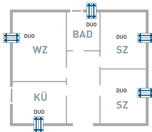
Einzelraumlüfter DUO mit Zu- und Abluft
