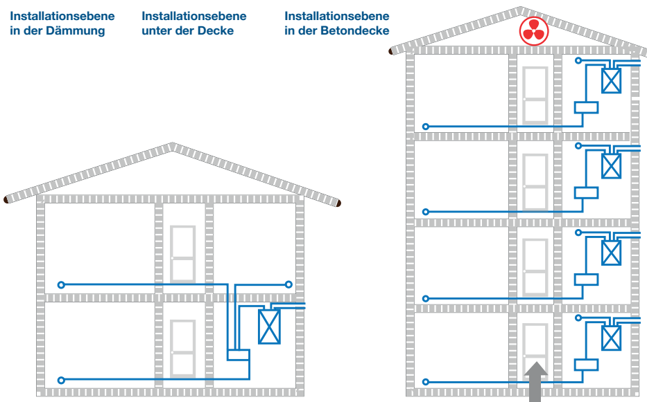
Einheitszentrales Einfamilienhaus / Zweifamilienhaus
